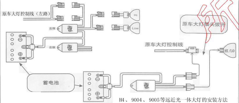
H4、9004、9005等远近光一体大灯的安装方法
